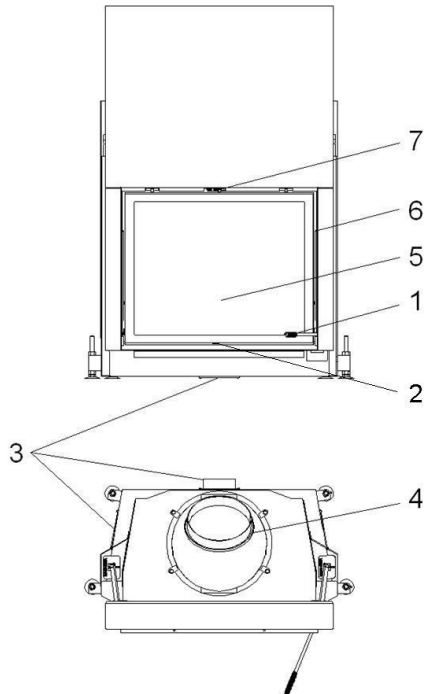
Bild. 1: Komponenter i Architektur-Kamine (schematisch)
